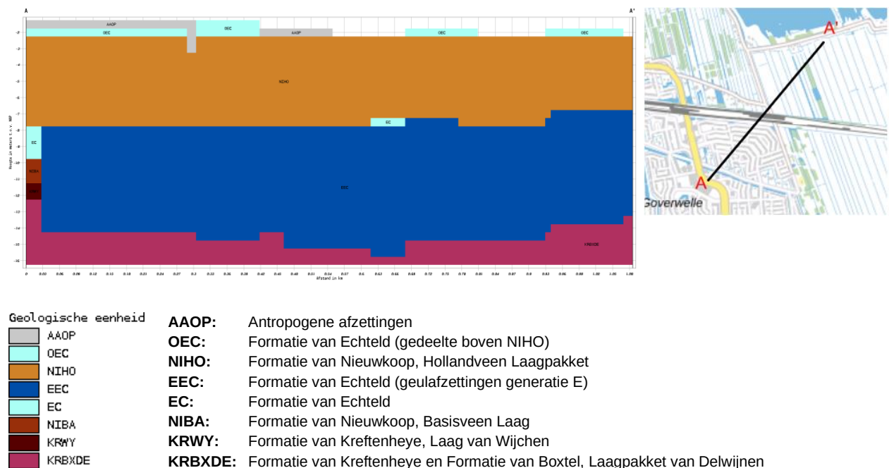
Figuur 1: Verticale doorsnede Achterwillensweg 146 te Gouda
