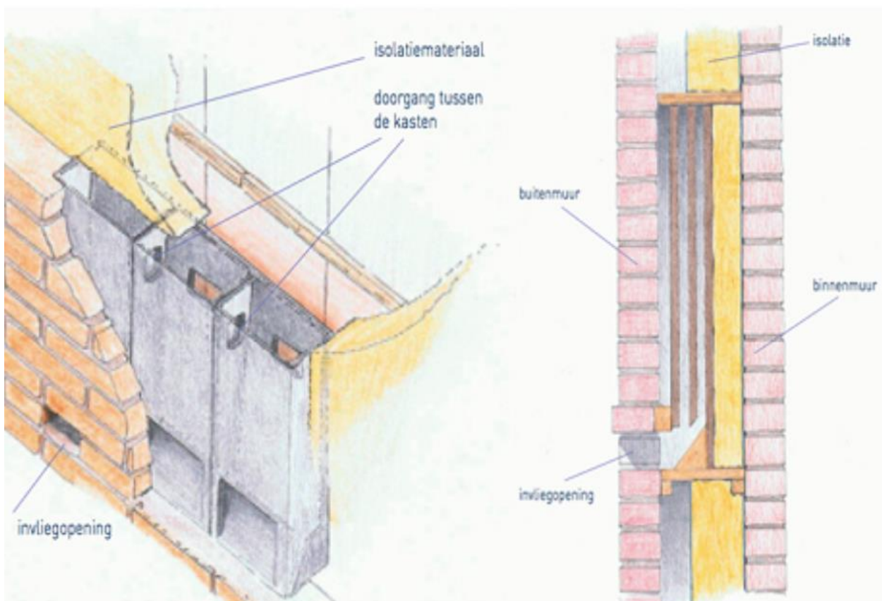
Afbeelding 11: Vrijwel onzichtbare inbouw van vleermuisstenen en technische informatie over de plaatsing daarvan.
