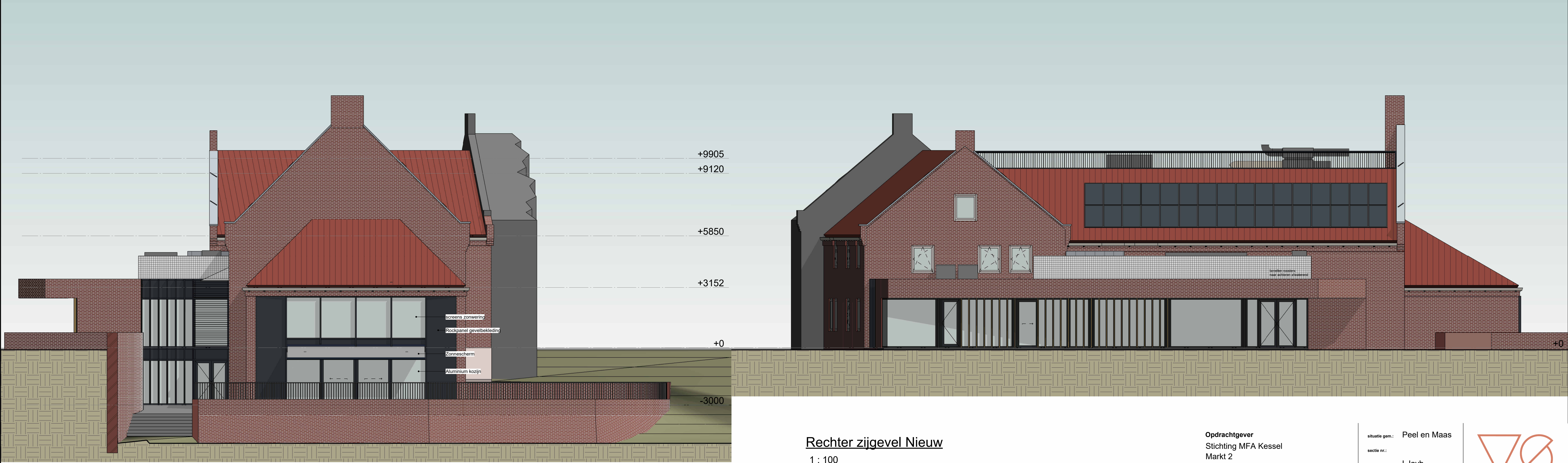
Achtergevel Nieuw 1 : 100
