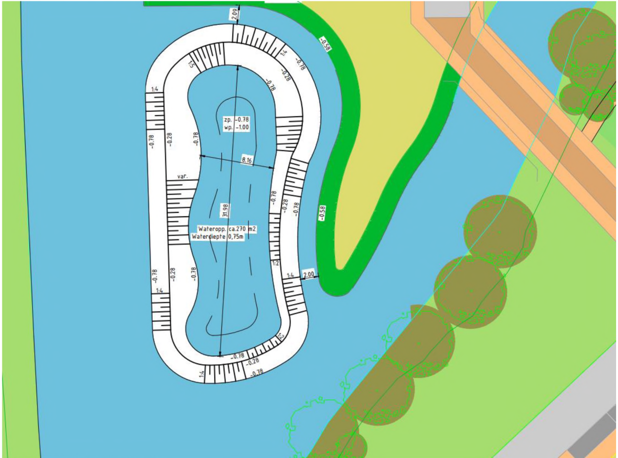
Tekening van een amfibieënpoel.
