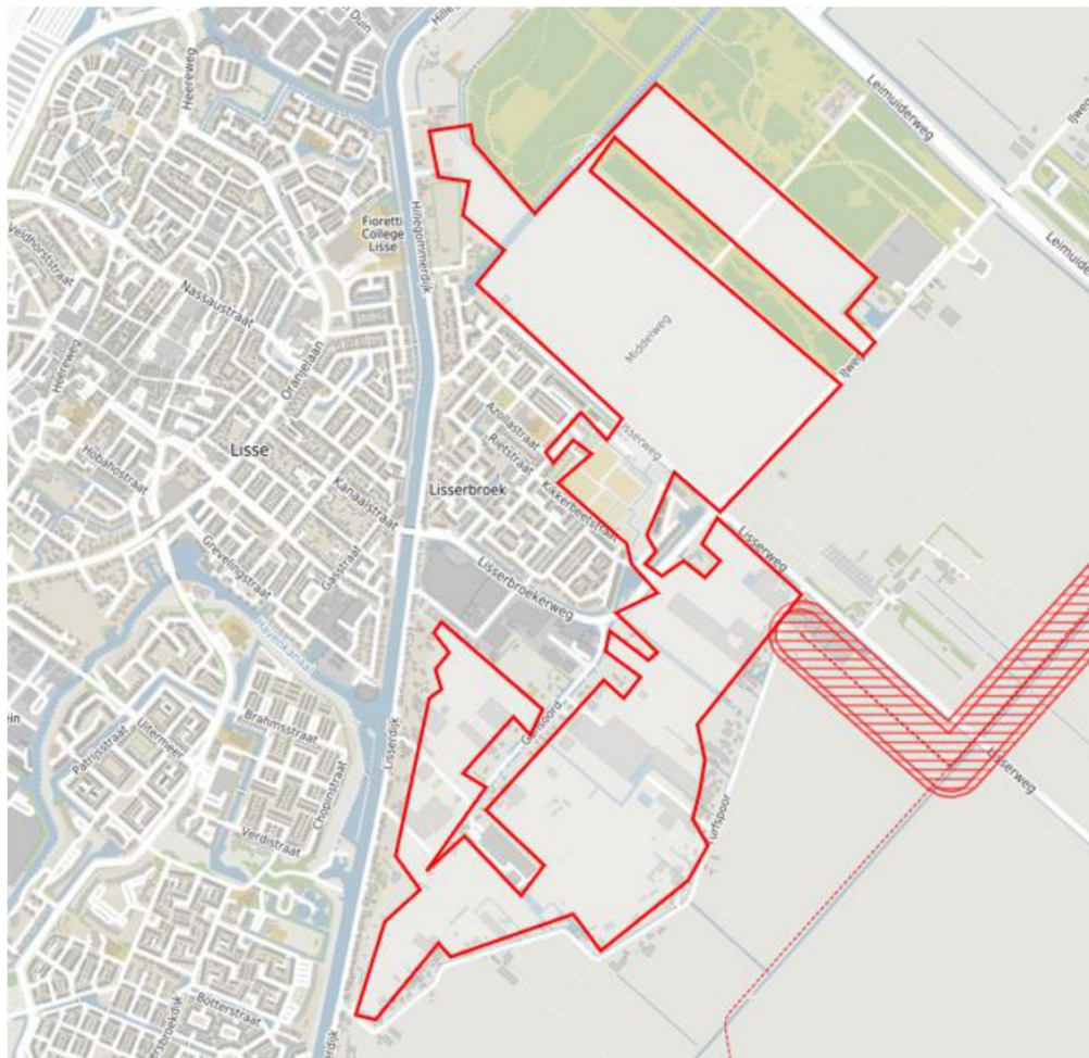
Figuur 5-39 Ligging van het brandaandachtsgebied van de buisleiding W-532-09 (rood gestreepte vlak)
