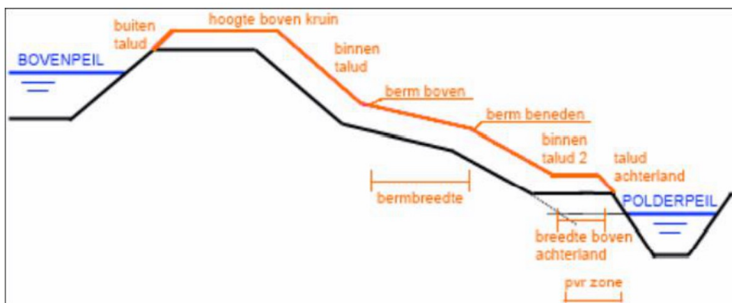
Figuur 5-76 Profiel van vrije ruimte (oranje lijn) (bron: Keur Hoogheemraadschap van Rijnland)
