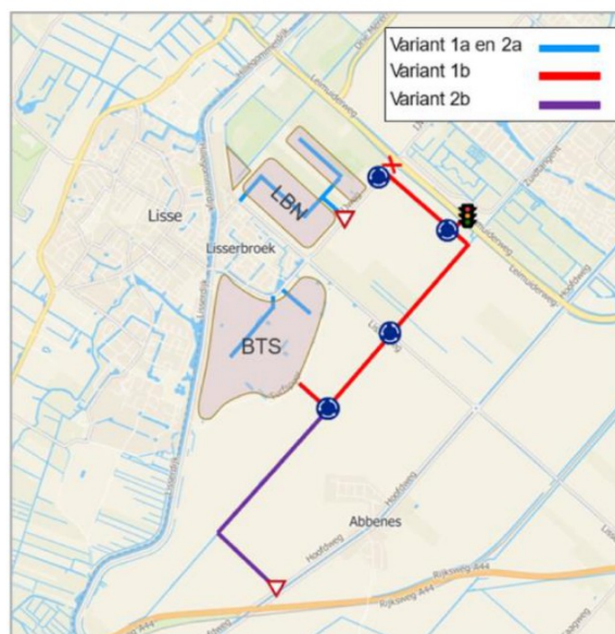
Figuur 3-6 Voorziene infrastructuur voor ontsluiting van Gebiedsontwikkeling Lissbroek met 4.000 woningen (voor uitleg varianten: zie paragraaf 3.4) (bron: Goudappel/Sweco, 2025)
