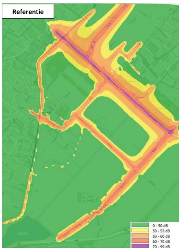
Figuur 5-26 Contouren wegverkeerslawaai referentiesituatie op 4,5 meter hoogte
