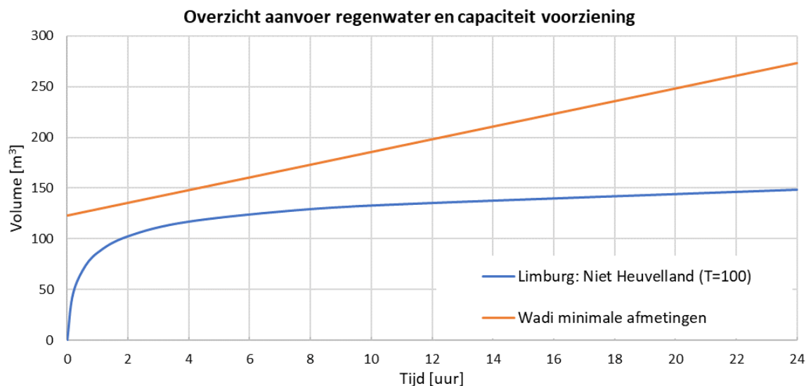
Figuur 5.2 Aan- en afvoercapaciteit wadi (minimale afmetingen)
