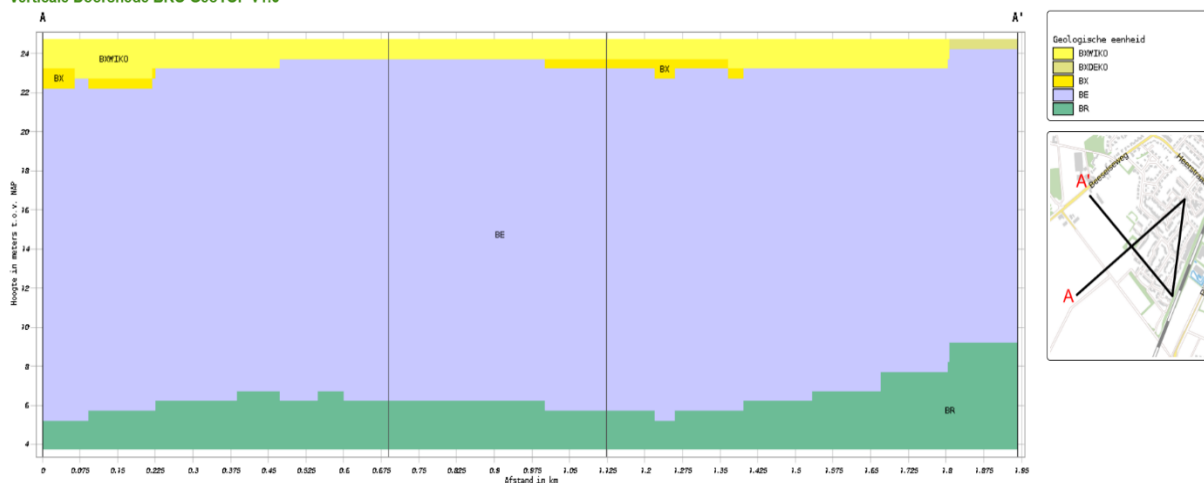
Figuur 3.1 Verticale doorsnede ondergrond BRO GeoTOP v1.6 [Bron TNO]
