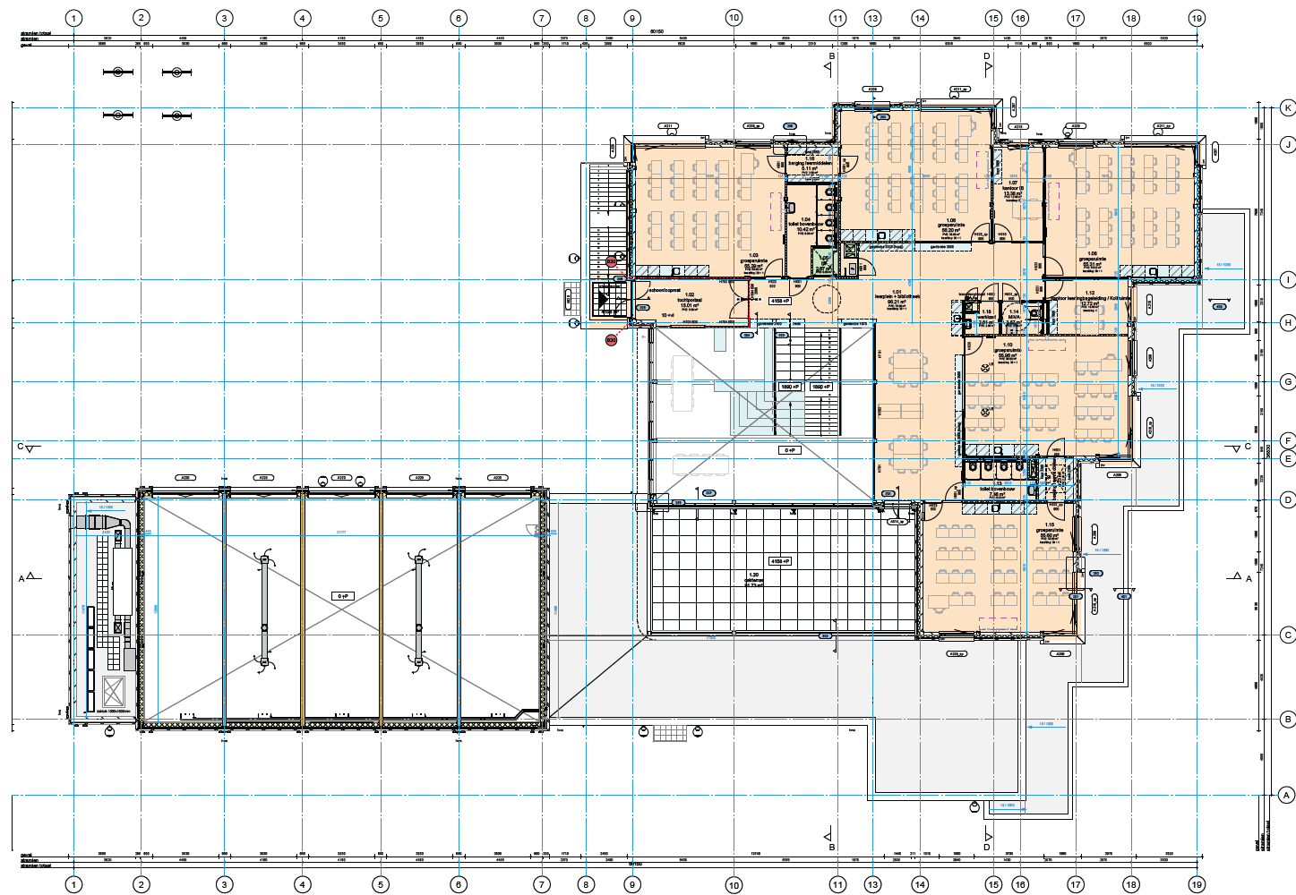
Eerste verdieping
