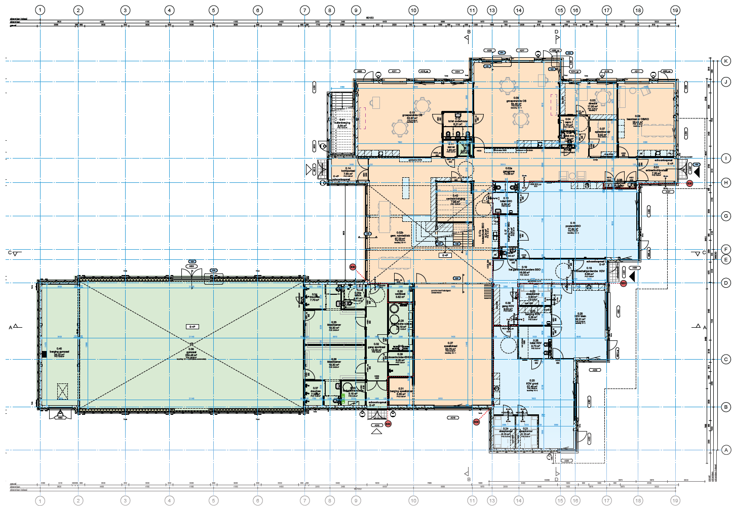
Begane grond
