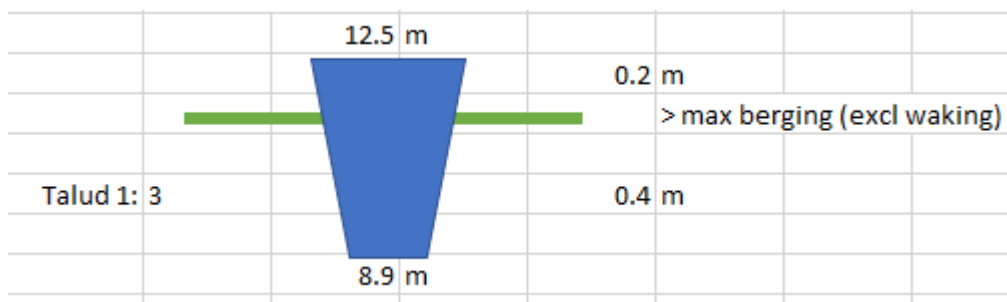
Figuur 4-3 Principeprofiel waterberging Wandelpad
