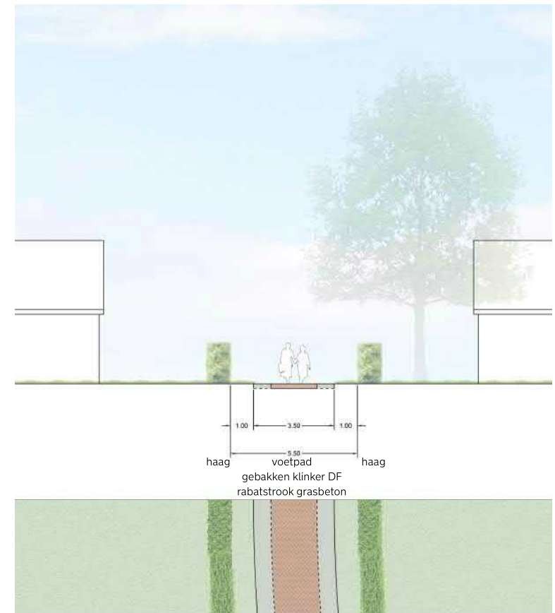
Profiel 7: Voetpad tussen erf en wijk
