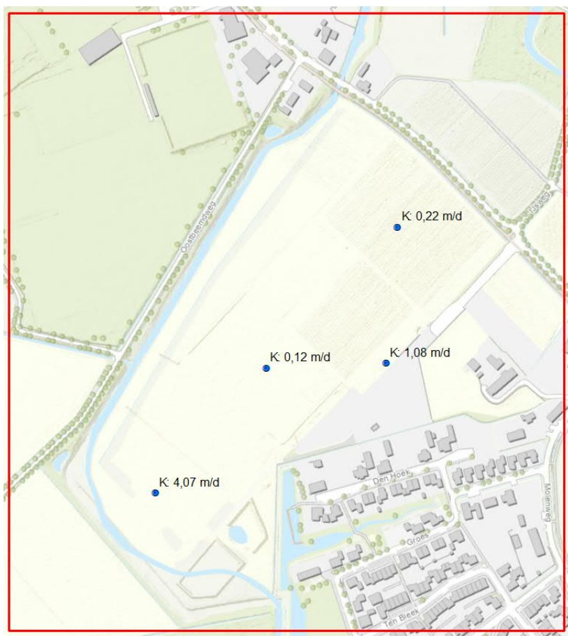
Figuur 2-9 Doorlatendheidsmetingen
