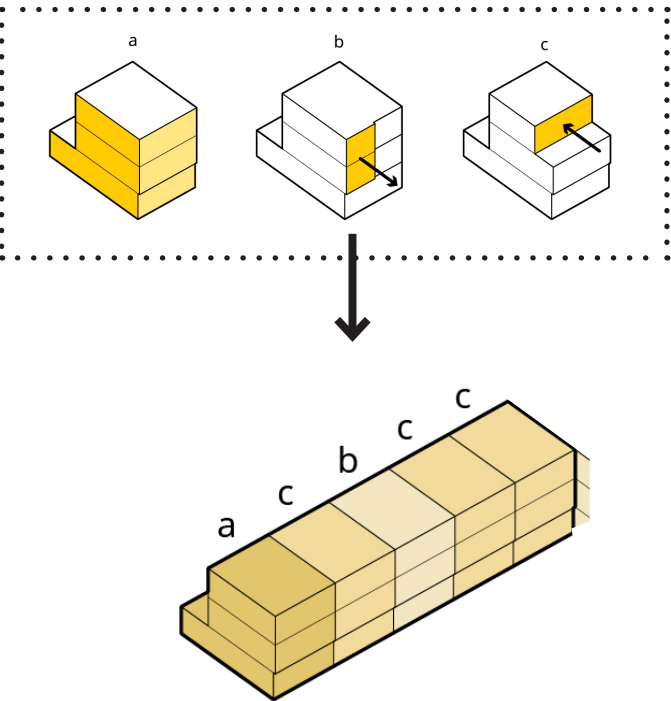
Differentiatie binnen de clusters door toepassen drie verschillende woningtypen.
