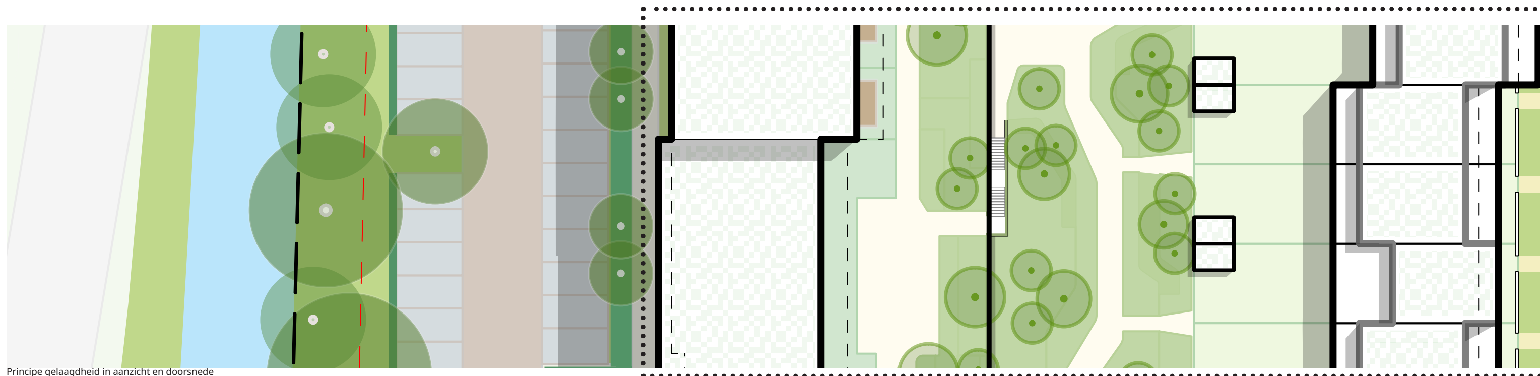
Principe gelaagdheid in aanzicht en doorsnede
