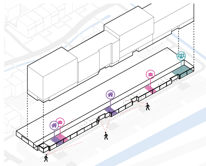
Functionele flexibiliteit in het plint. Ruimte voor woon-werk units en individuele entrees.
