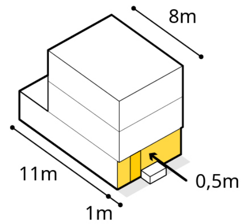
Basis zuidkant: kleine inpandige setback van 0,50 mtr. met een stoep van 1.0 mtr. als voorzone
