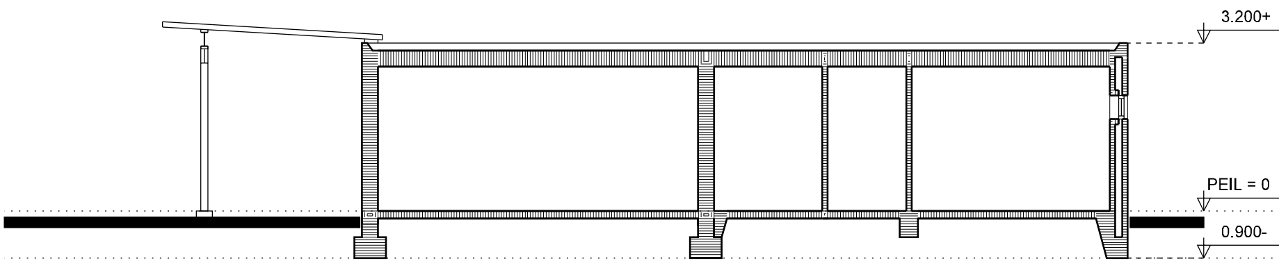
Doorsnede A-A
