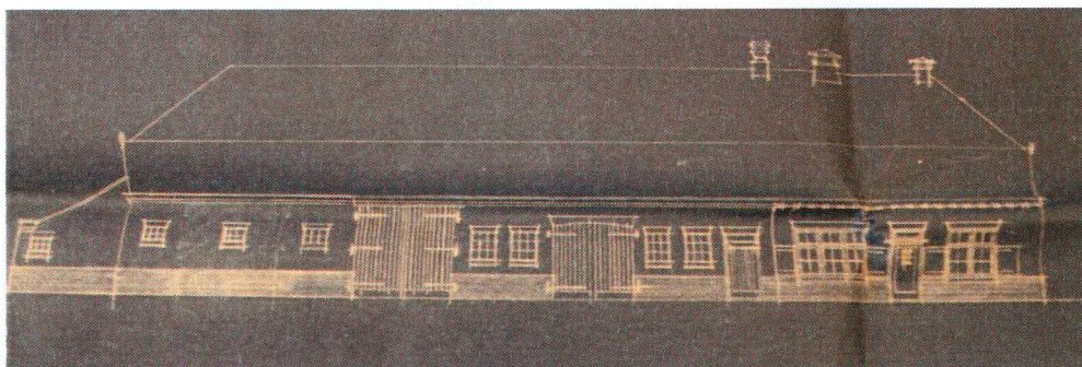
Voorgevel, uitsnede van de bestektekening. Bron: BHIC, 1504-1531.
