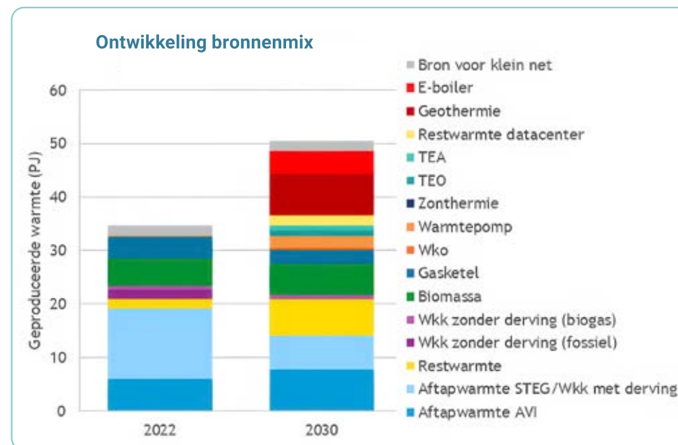
Figuur 17: Warmteproductie voor de warmtenetten in 2022 en verwachting 2030. Bron: Rapport 'Verduurzaming bronnen voor warmtenetten', 2023, CE Delft
