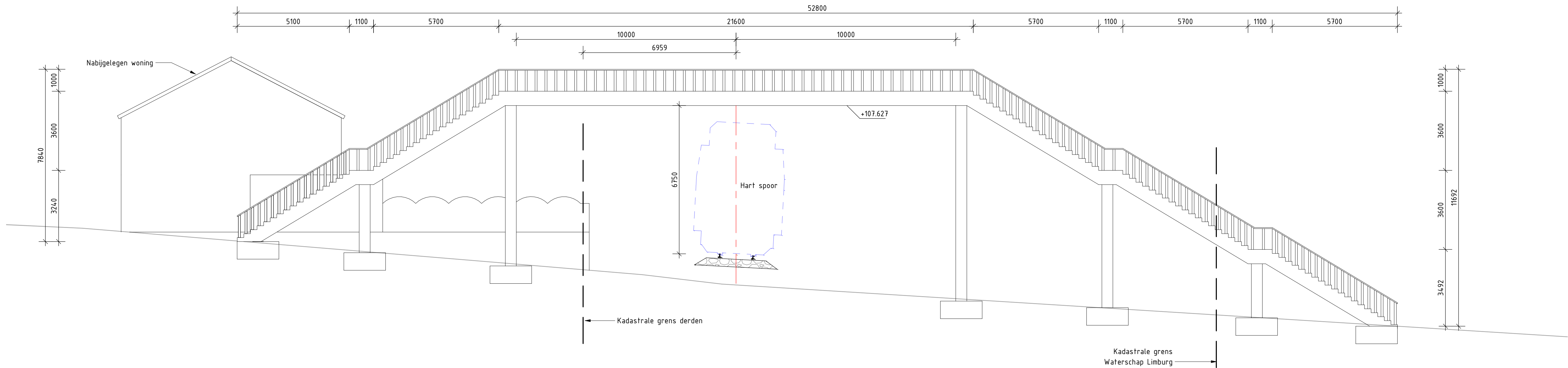
Langsdoorsnede A Schaal: 1 : 100
