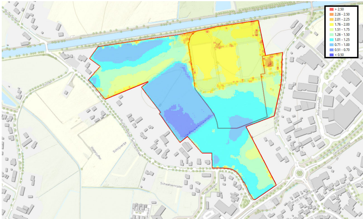
Figuur 2.11 Berekende ontwateringsdiepte tijdens GHG [m].
