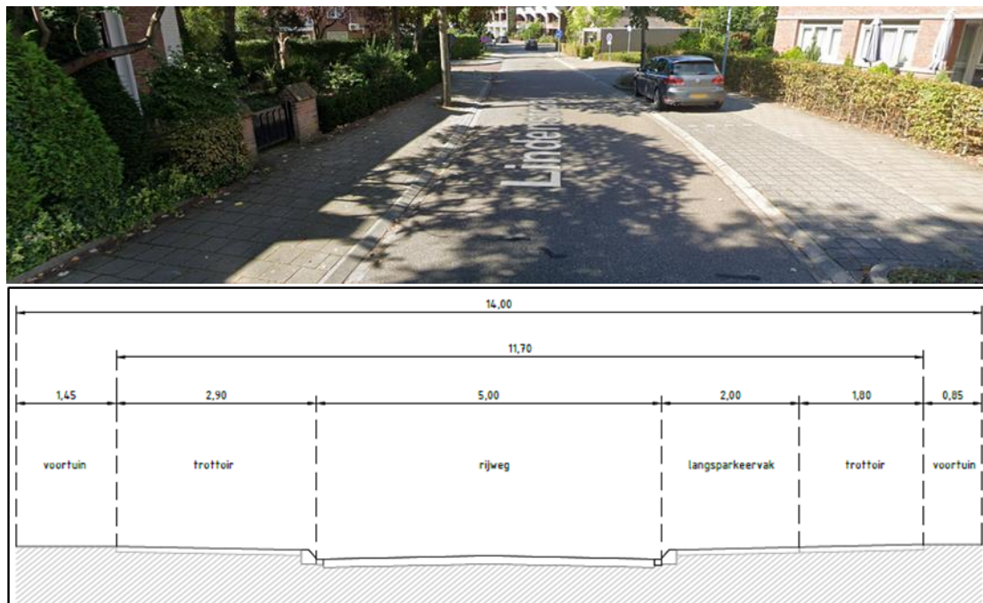
Figuur 28: Dwarsprofiel traject 5 ter hoogte van Lindenstraat 2
