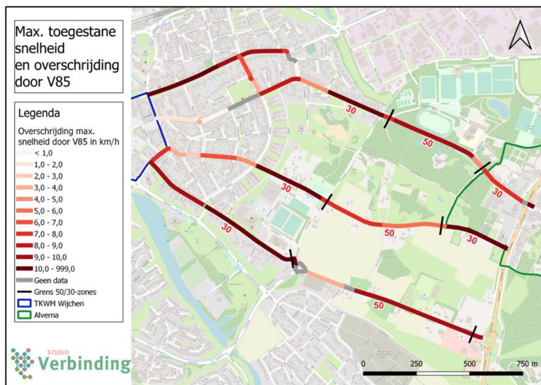
Figuur 5: Maximum snelheden en overschrijding hiervan door de V85 in km/uur..
