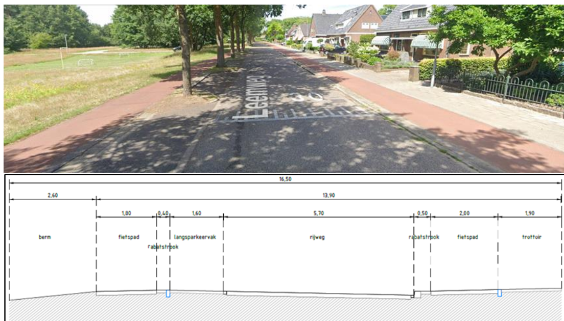
Figuur 26: Dwarsprofiel traject 3 ter hoogte van Leemweg 81
