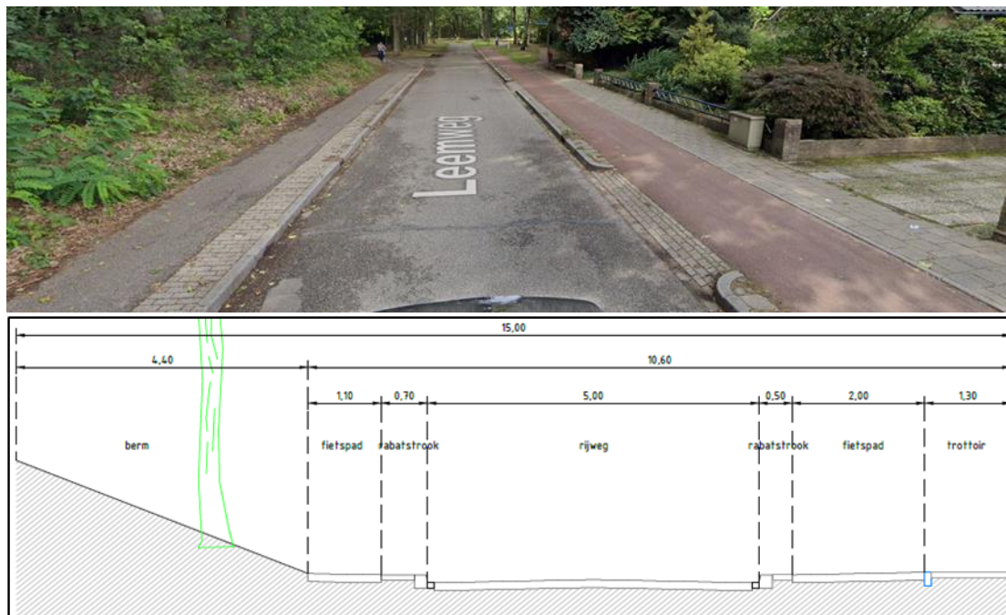
Figuur 24: Dwarsprofiel traject 1 ter hoogte van Leemweg 125
