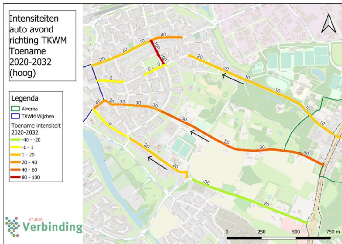
Figuur 67: Toename intensiteiten avondspits in verkeersmodel richting TKWM
