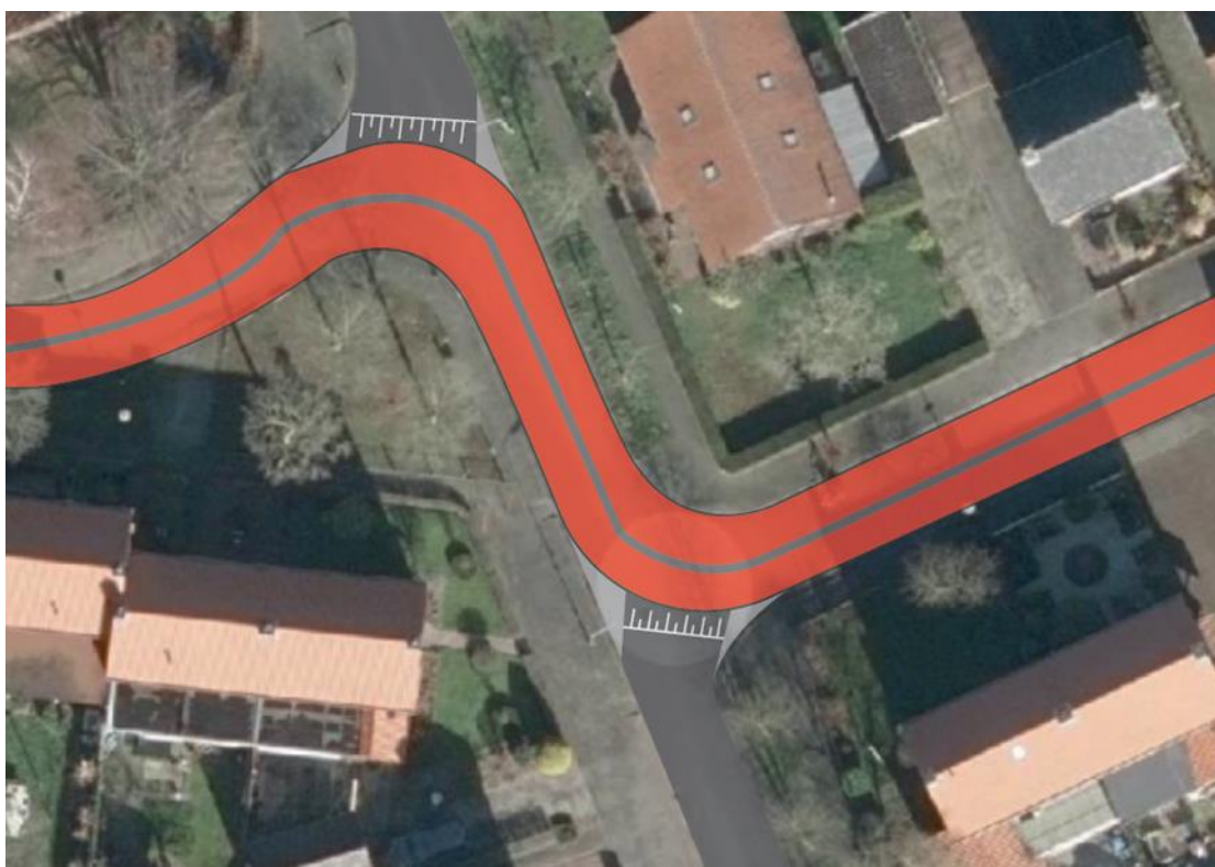
Figuur 57: Boveaanzicht fietsstraat traject 5 bij bajonet kruispunt met de Meidoornstraat
