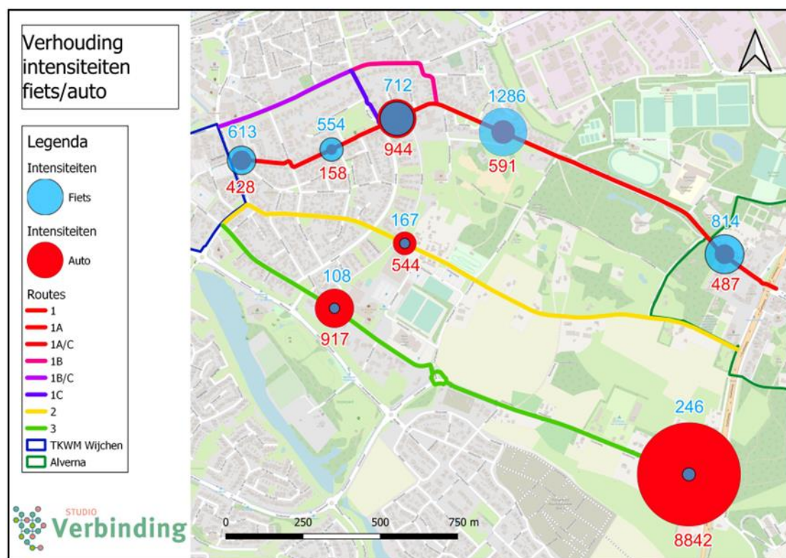
Figuur 3: Visualisatie van de verhouding in intensiteiten tussen de auto en fiets per tellocatie
