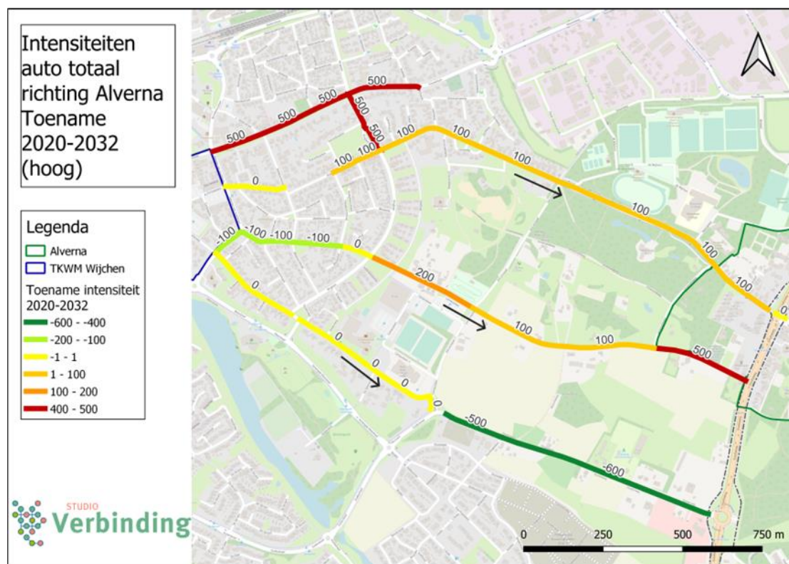
Figuur 62: Toename intensiteiten in verkeersmodel richting Alverna
