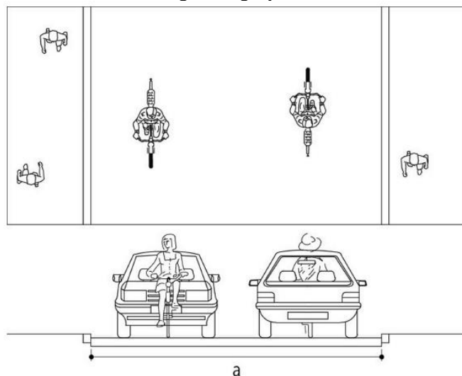
a) Rijbaanbreedte 4,50 meter
