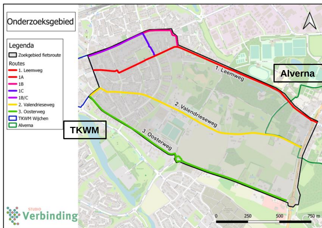
Figuur 1: Onderzoeksgebied hoogwaardige fietsroute Alverna - TKWM
