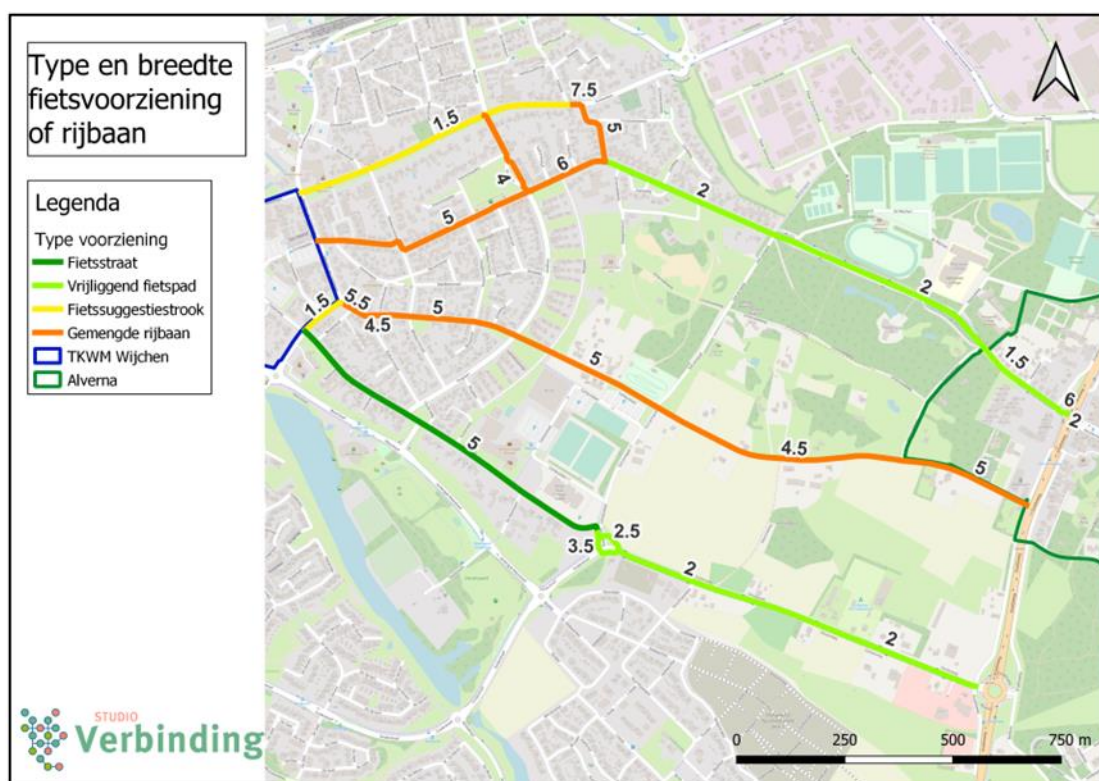
Figuur 20: Soort/type fietsvoorziening en de breedte ervan.
