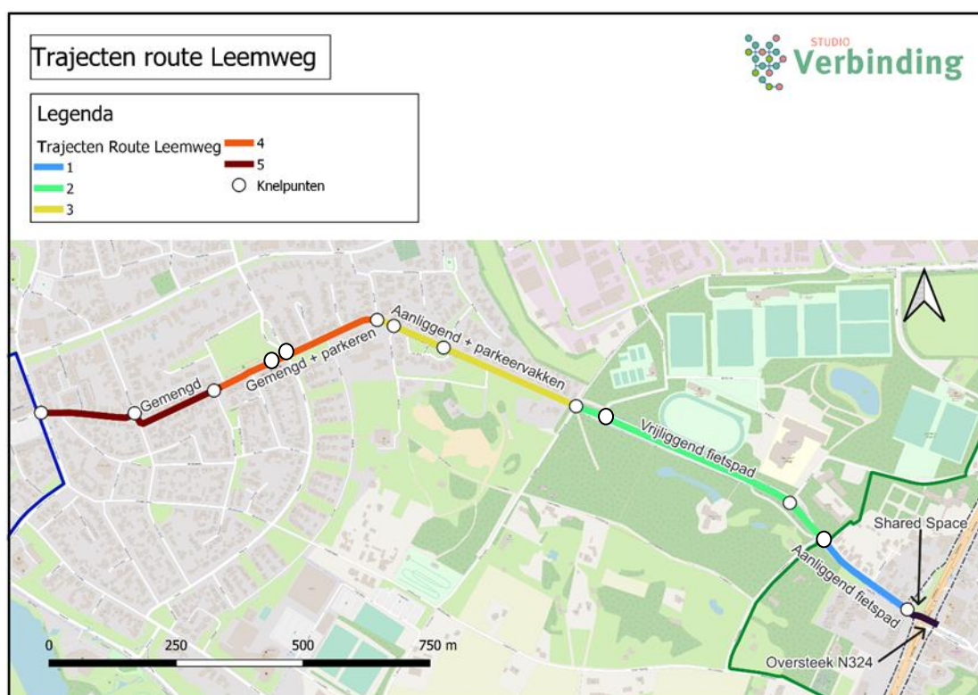
Figuur 23: Opsplitsing route in vijf trajecten
