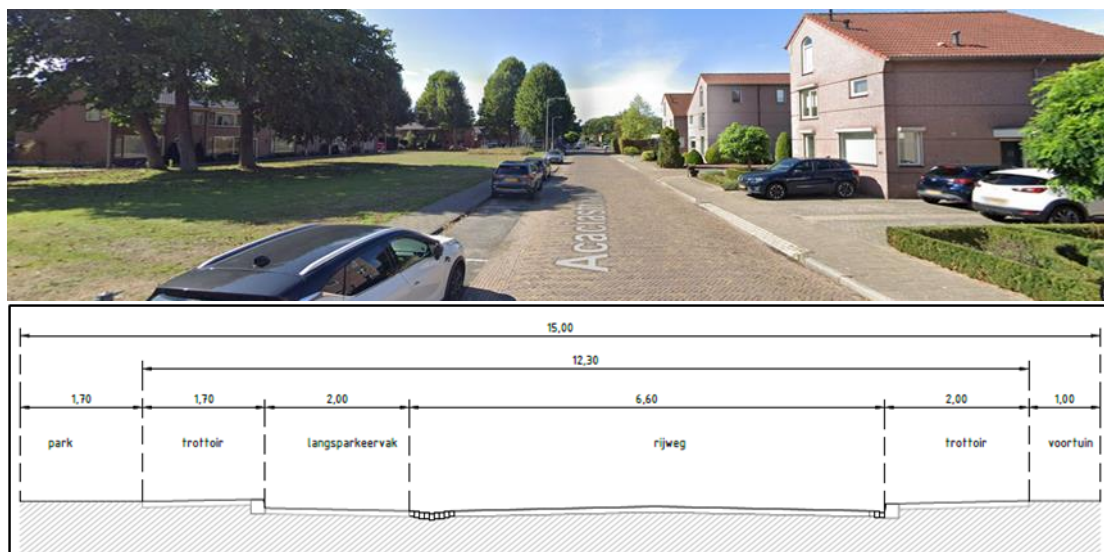
Figuur 27: Dwarsprofiel traject 4 ter hoogte van Acaciastraat 49
