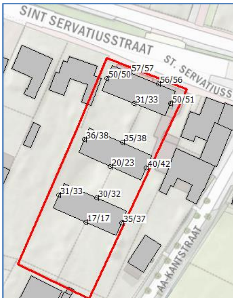
Afbeelding 6. Geluidbelastingen L_{den} Gemeentewegen Berekende geluidbelastingen op een hoogte van 2,0 ; 5,0 meter
