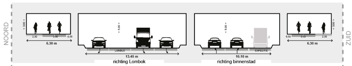
Huidige indeling Daalsetunnel.
