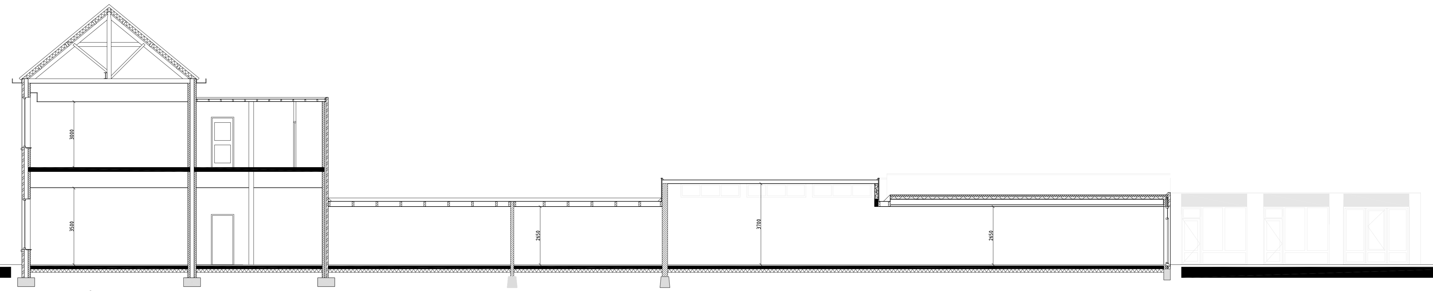
Doorsnede A
