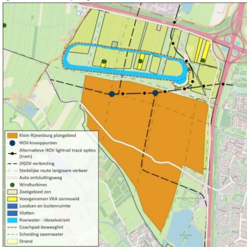
Figuur 6.2: ideaalvariant inpassing roeiwater
