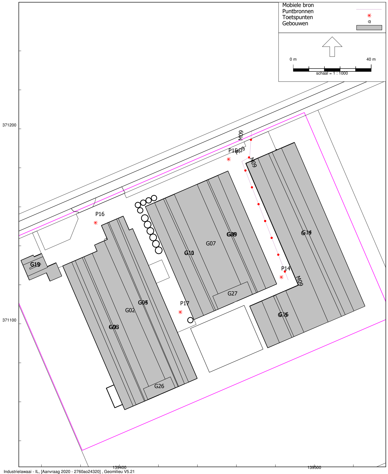
Figuur 4.4 Overzicht geluidbronnen Tractor/shovel
