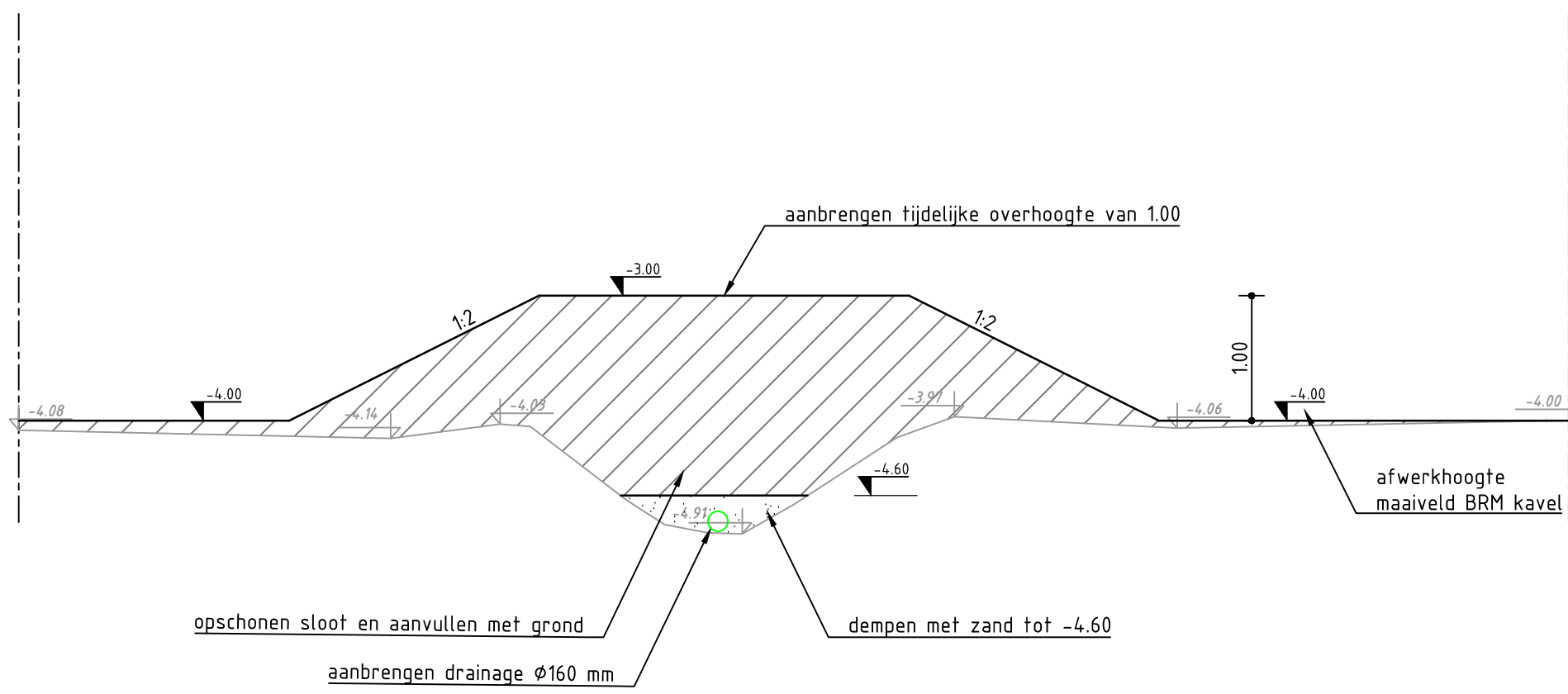
N.A.P. -7.00 Dwarsprofiel B-B SCHAAL 1 : 50
