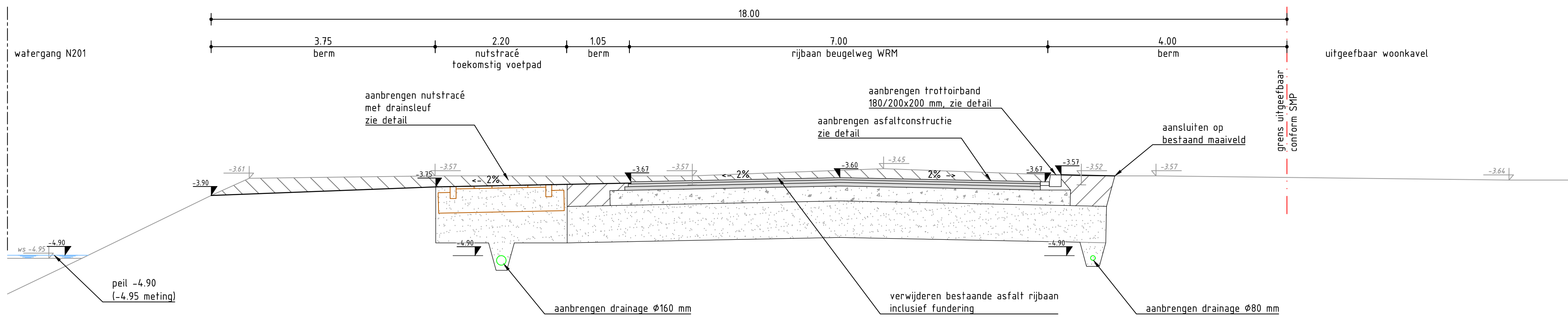
N.A.P. -7.00 Dwarsprofiel D-D SCHAAL 1 : 50
