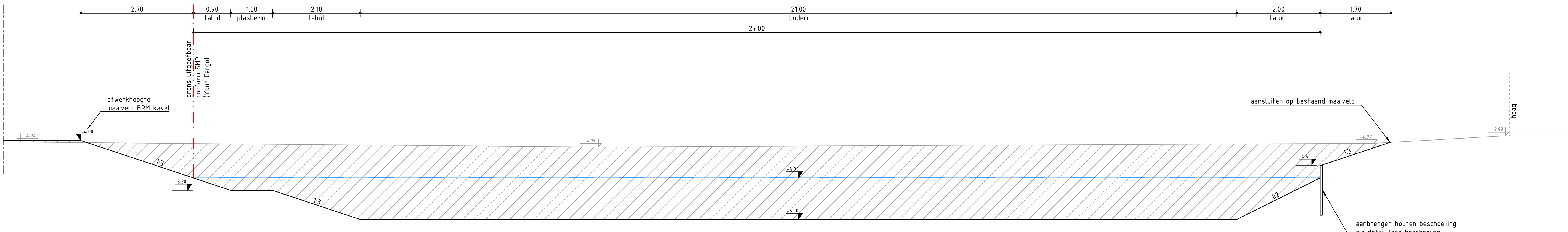
N.A.P. -7.00 Dwarsprofiel F-F SCHAAL 1 : 50
