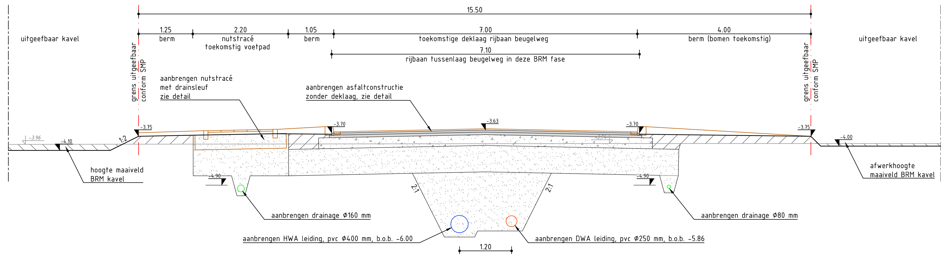
N.A.P. -7.00 Dwarsprofiel E-E SCHAAL 1 : 50
