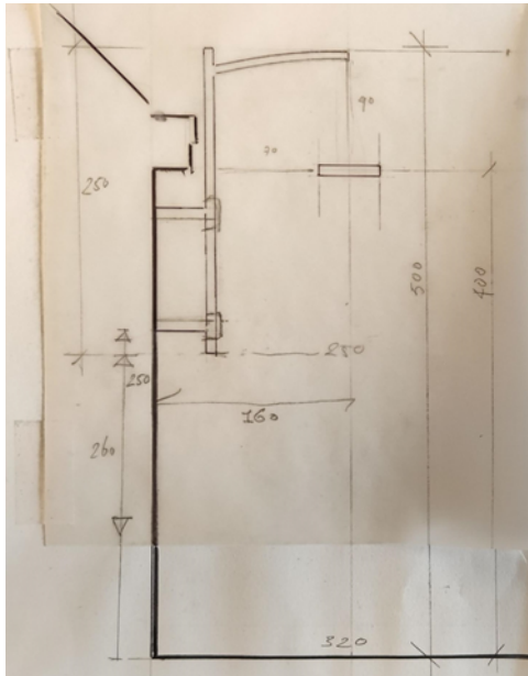
Figuur 8: Bevestiging lichtstrook overzijde Haniahof
