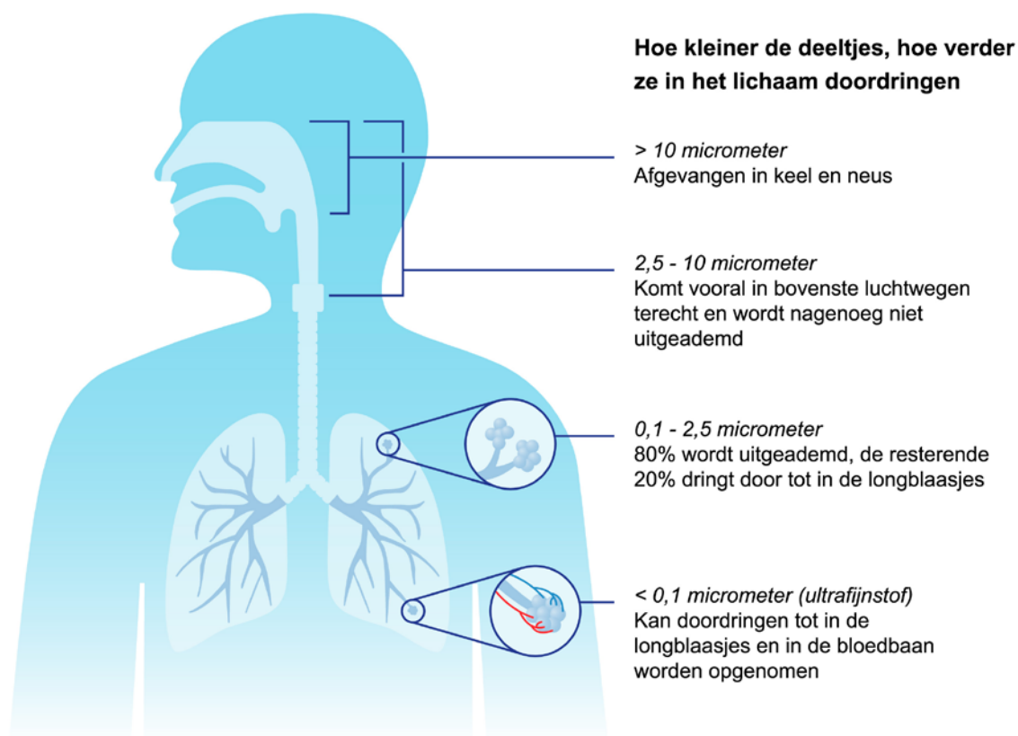
Figuur B2.2 Deeltjesgrootte en tot waar deze het lichaam binnendringen (Gezondheidsraad, 2018).
