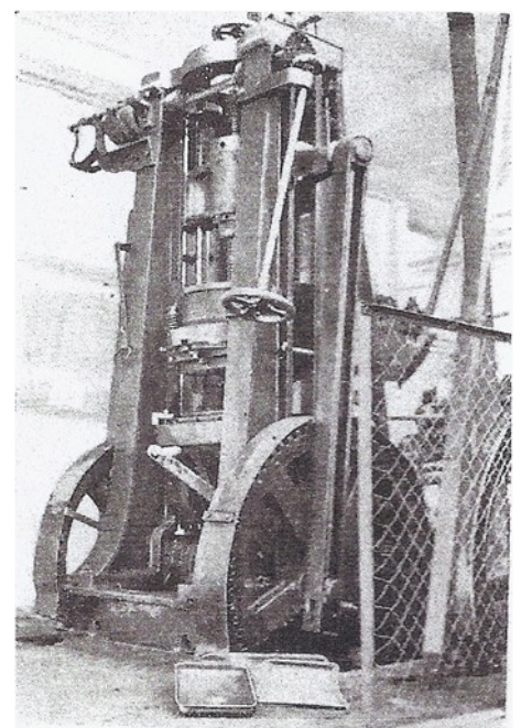
100 tons metaalpers
