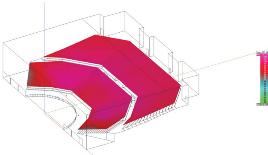
Voorbeeld SPL direct niveaueverschil (voorbeeld met line-array)
