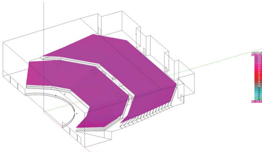
Voorbeeld SPL total niveaueverschil (voorbeeld met line-array)
