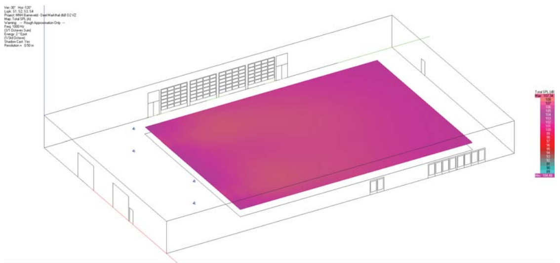
Voorbeeld SPL total niveaoverschil (voorbeeld met line-array)
