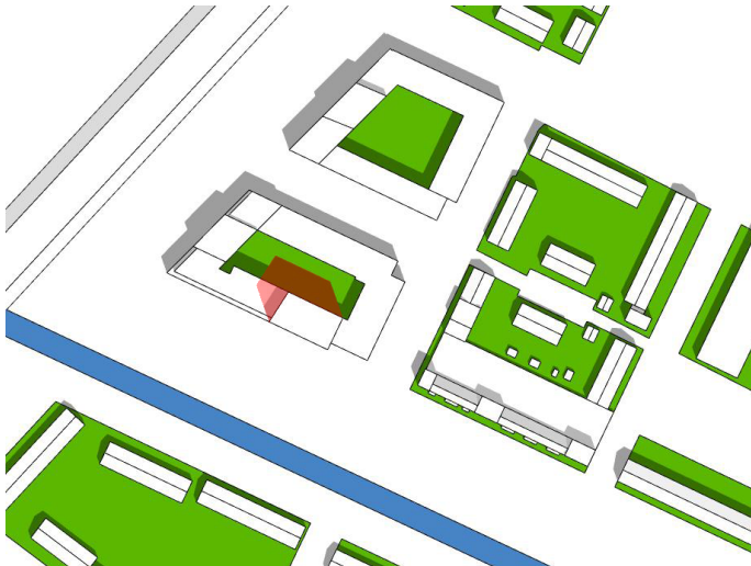
21 juni 12.00 - met hoogteaccent
