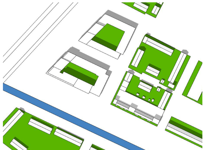
21 juni 14.00 - zonder hoogteaccent
