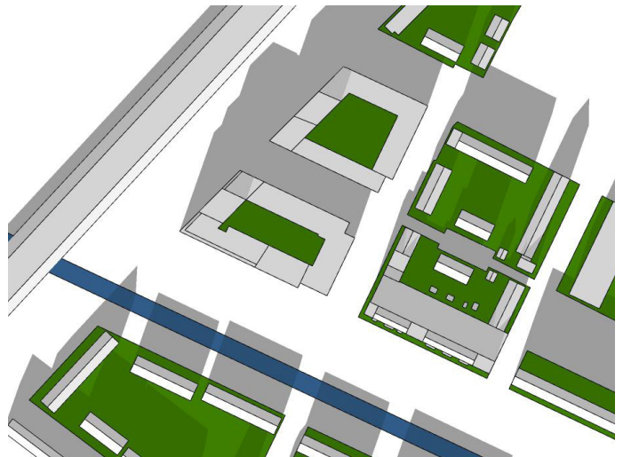
21 december 14.00 - zonder hoogteaccent
