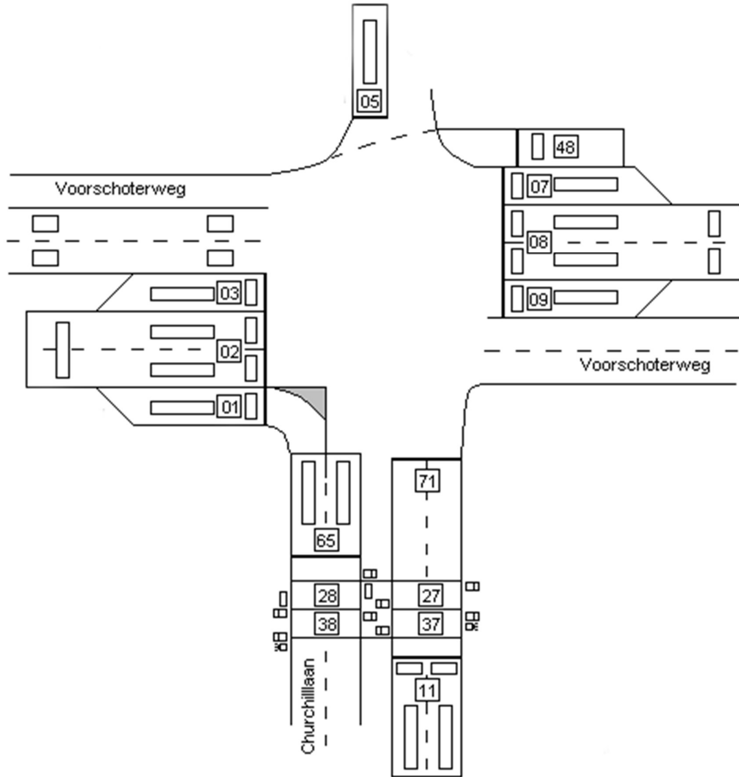
Figuur 1: Kruispuntconfiguratie VRI 0608
