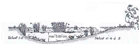
Doorsnede wadi
