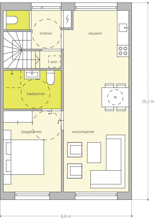
begane grond
