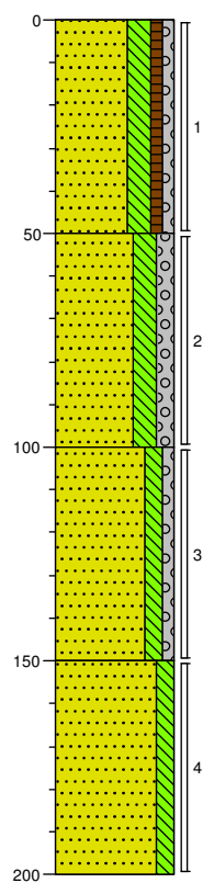
Gat/boring:A13
