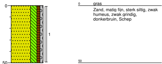
Gat/boring:A03
