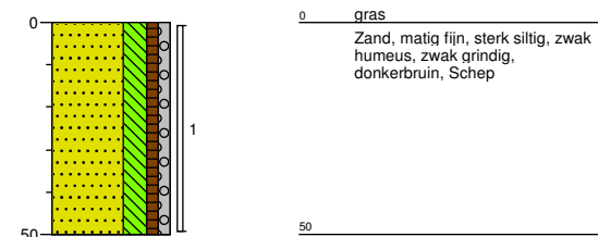
Gat/boring:A06
