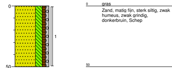
Gat/boring:A04
