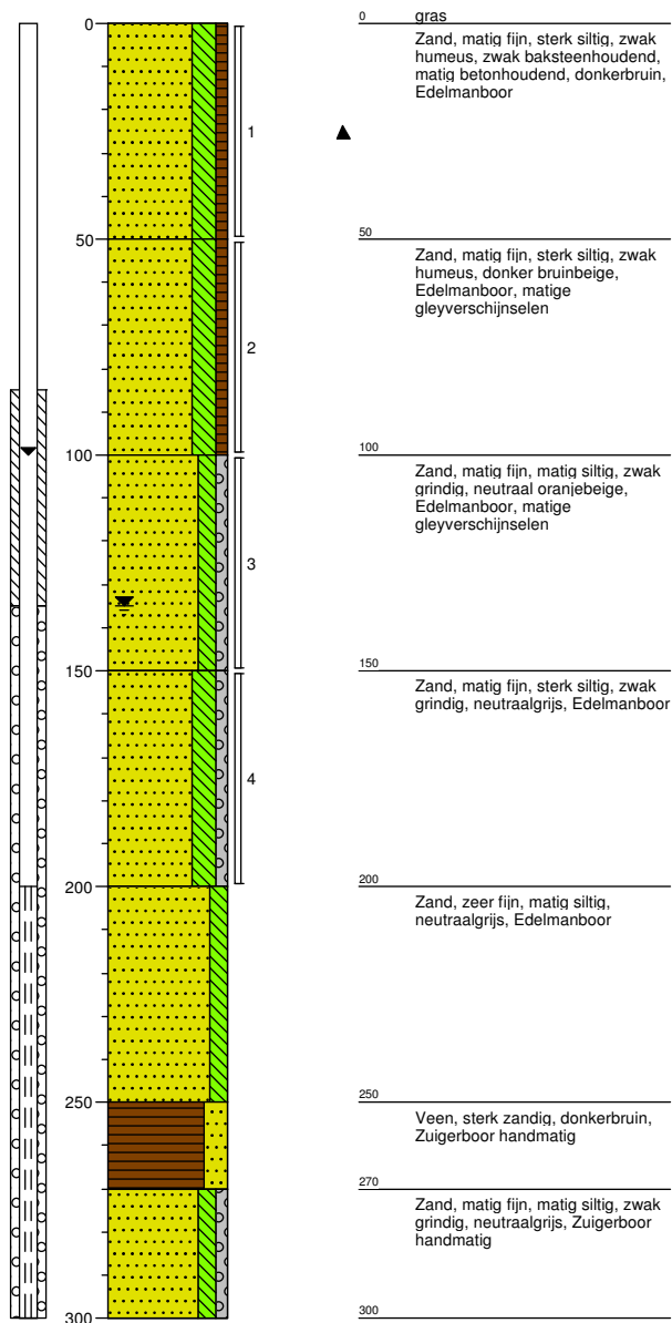
Gat/boring:B01
