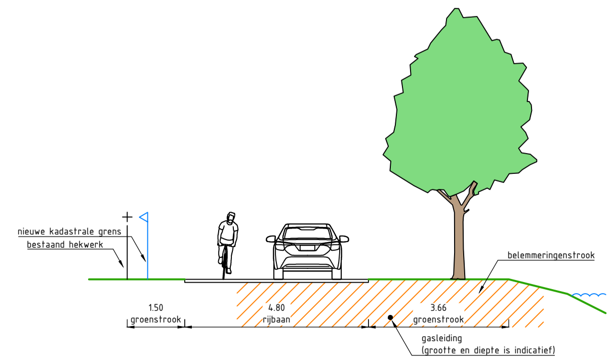
Dwarsprofiel A-A Schaal 1:100
