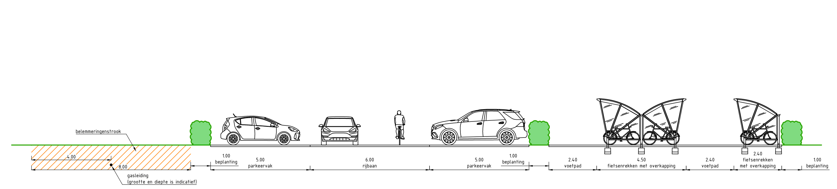
Dwarsprofiel B-B Schaal 1:100
