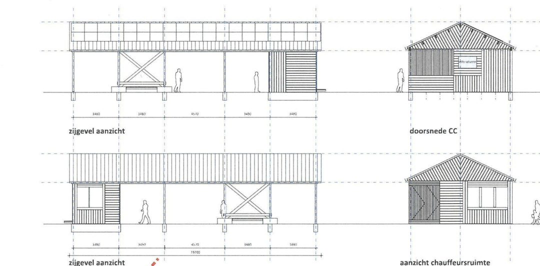
zijgevel aanzicht
