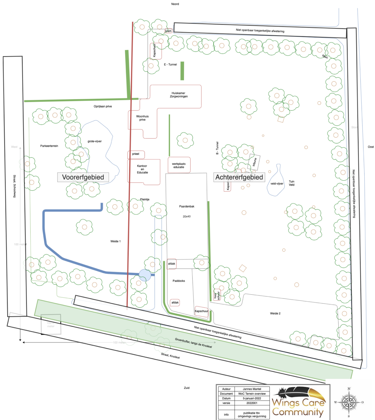
Figuur 1: Plattegrond voor en achtererf gebied versie 2022001
