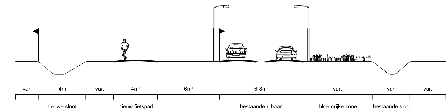
Nieuw profiel - N625 - John F. Kennedybaan
