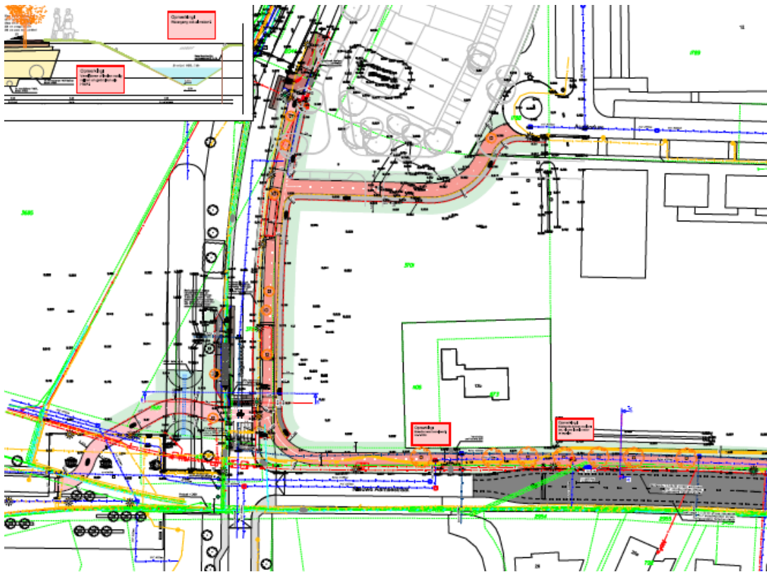
Schetsontwerp fietspad Nieuwe Aamsestraat oostzijde bij fietsonderdoorgang
