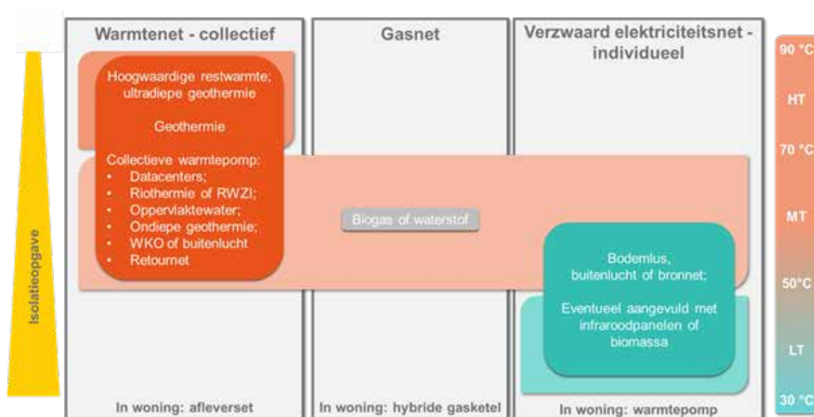
Figuur 6: energie-infrastructuren met bronnen en benodigde systemen in de woning. De kolom rechts toont welke afgiftetemperaturen horen bij warmte-optie, die rechtstreeks is gekoppeld aan de isolatieopgave (kolom links)
