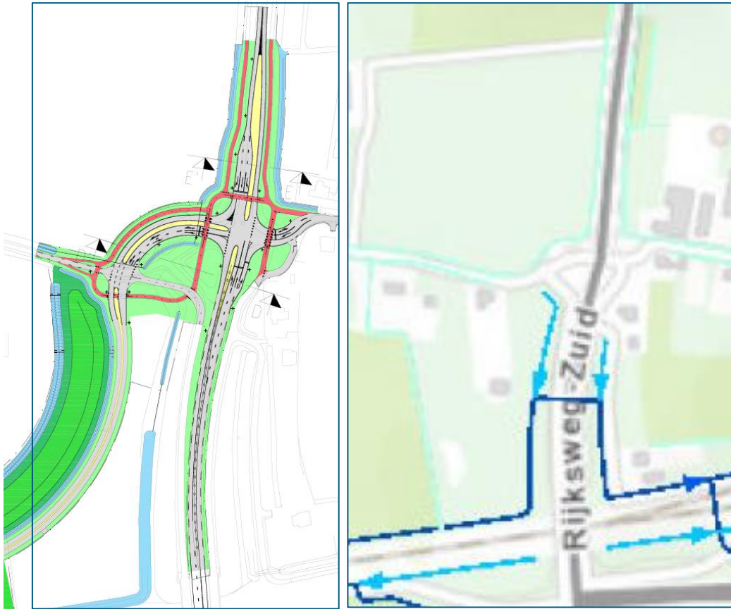
Figuur 8 Ontwerp kruising Rijksweg-Zuid / Ontsluitingsweg
