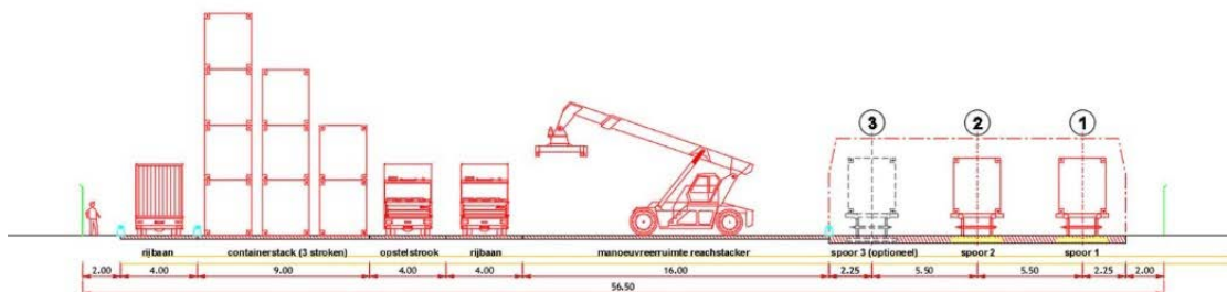
Figuur 4.7 Principeddoorsnede Zuidvariant (van zuid naar noord)
