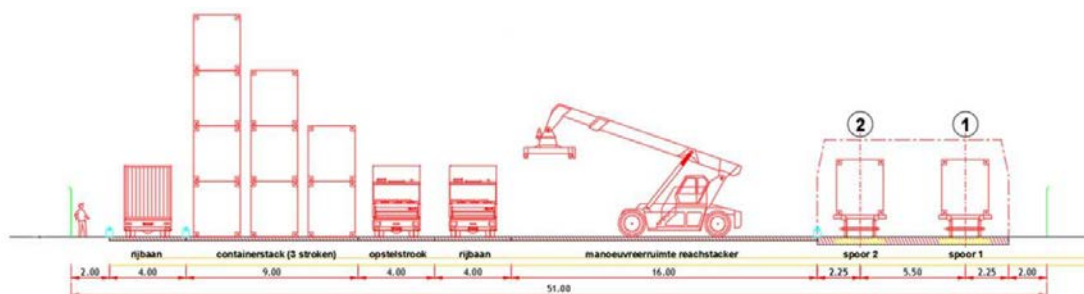
Figuur 4.3 Principeddoorsnede van de RTG, weergegeven van noord (links) naar zuid (rechts)
