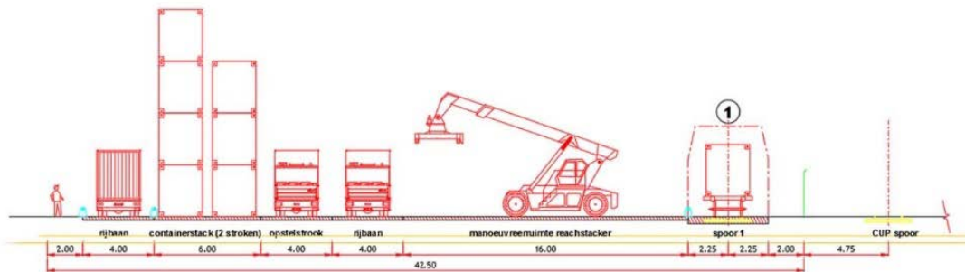
Figuur 4.6 Principeddoorsnede Middenvariant (van noord naar zuid)
