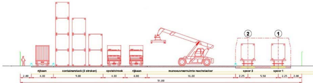
Figuur 4.5 Principeddoorsnede Noordvariant (van noord naar zuid)
