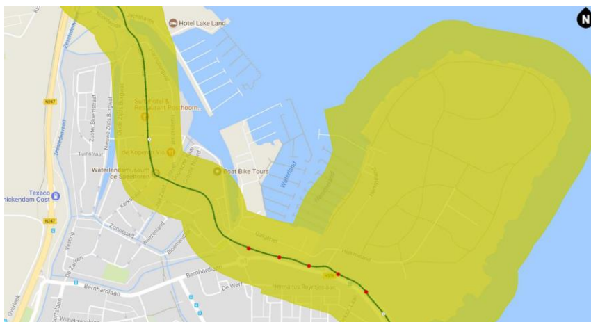
figuur 4.1: Beschermd zone door de waterkering (groen).
