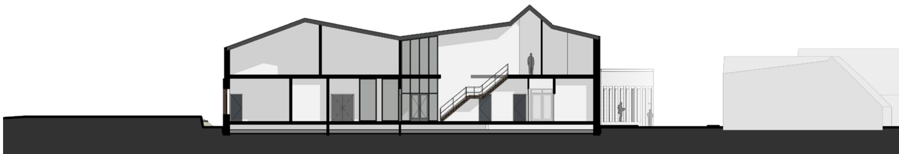
DOORSNEDE B-B
