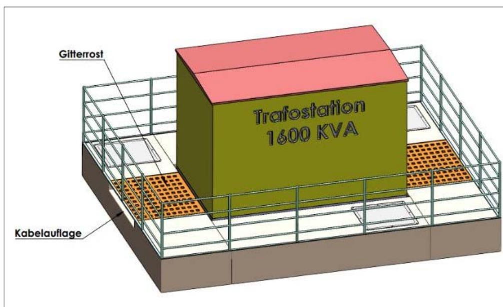
Figuur 11. Schematische weergave trafostation bovenwater (kleurstelling wordt blauw/grijs).
