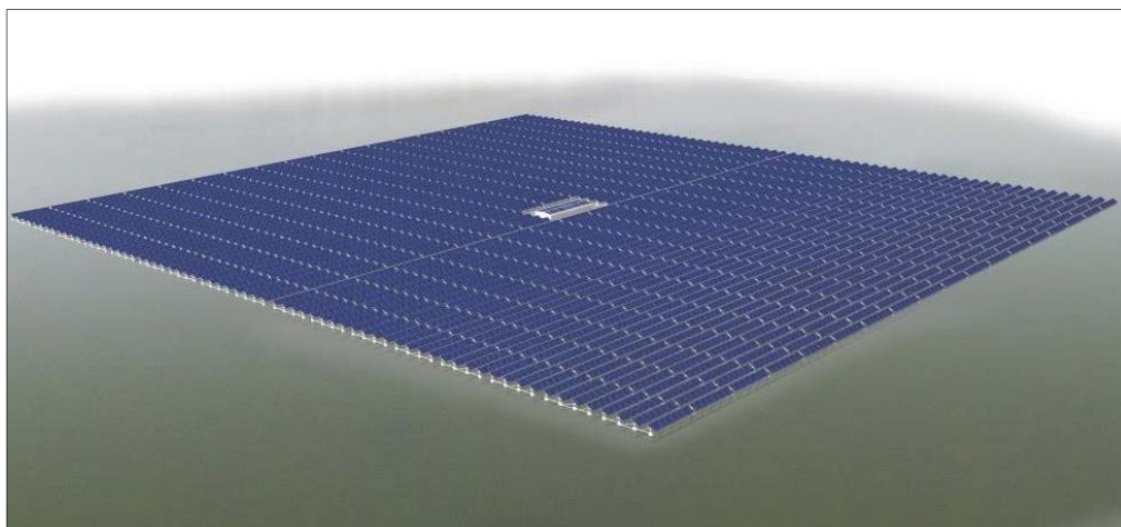
Figuur 10. Visualisatie module met betonnen bak.
